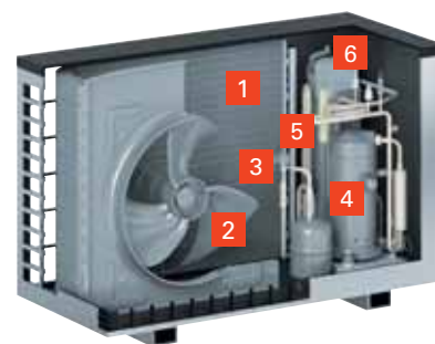
VITOCAL 200-A Außeneinheit
